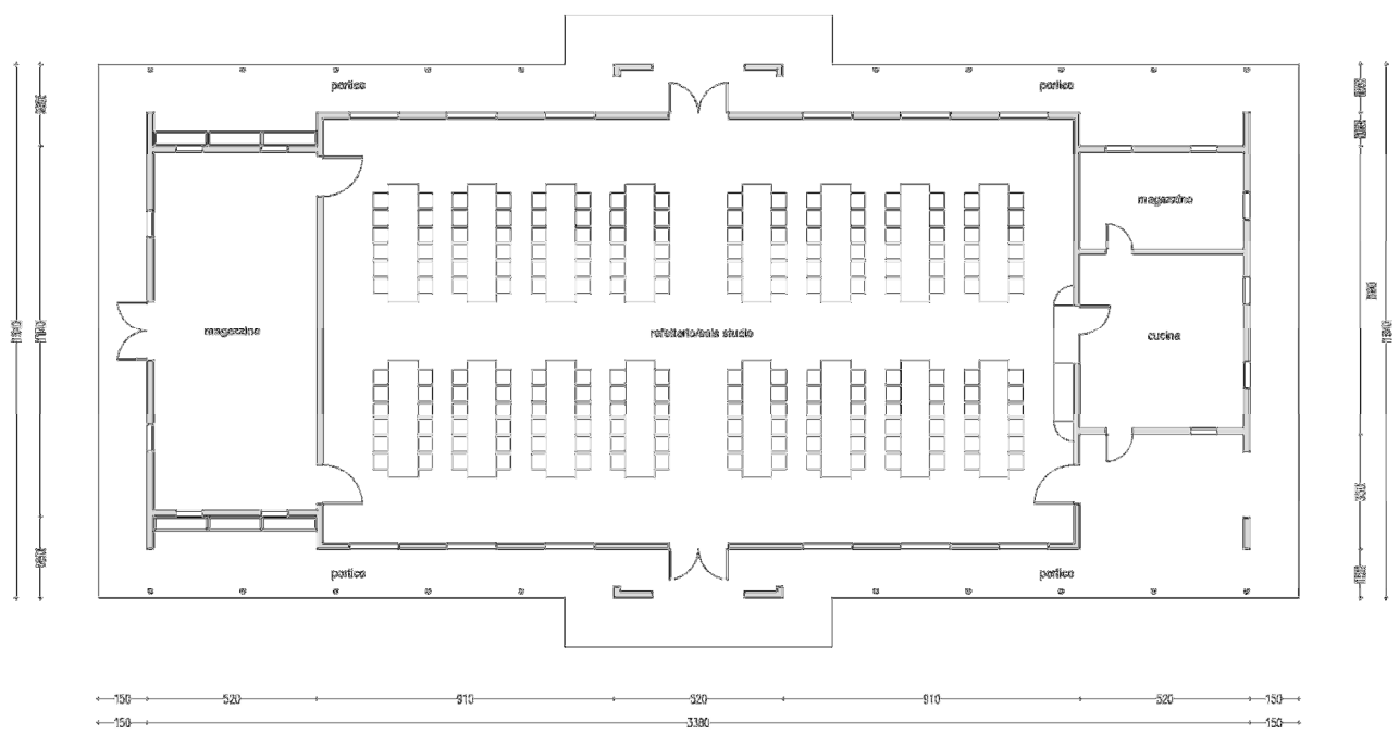
Sala polifunzionale - Planimetria di progetto
