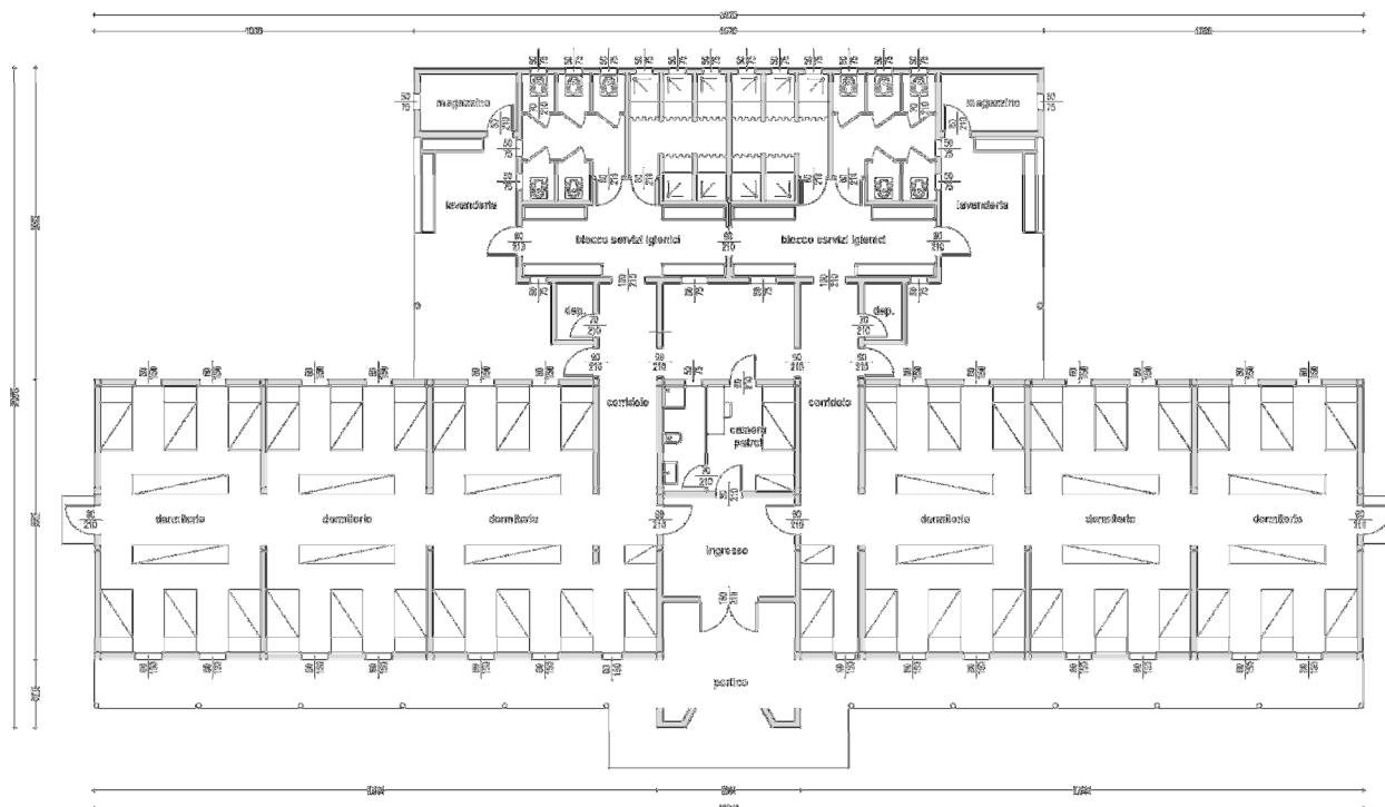
Dormitorio per Bambini - Planimetria di progetto
