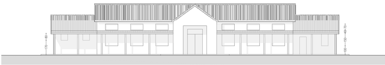
Prospetto principale
